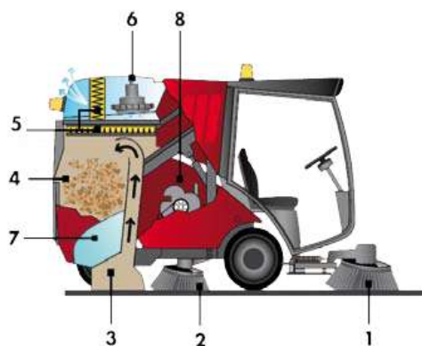
1 Cepillos delanteros | 2 Cepillos laterales | 3 Boca Aspirante | 4 Contenedor de residuos | 5 Filtros | 6 Turbina aspirante | 7 Depósito de Agua | 8 Motor
